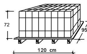
Dimensioni bancale
