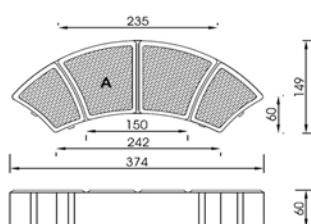
Elementi per mq. n° 27 - Pezzi per strato n°14 mod A, n°14 mod B
