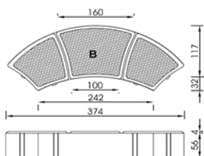
Elementi per mq. n° 27 - Pezzi per strato n°14 mod A, n°14 mod B
