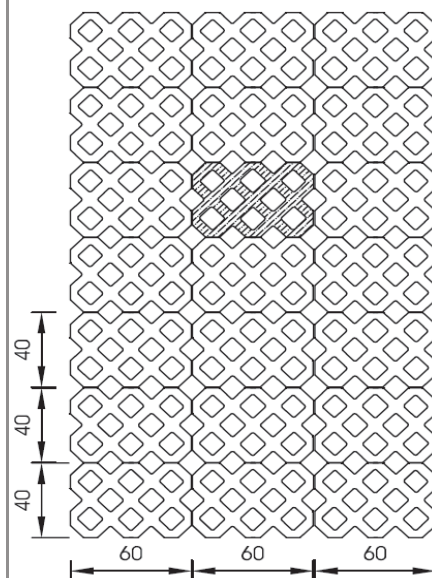
Normale a giunti continui (possibilità di posa con pinza meccanica)
